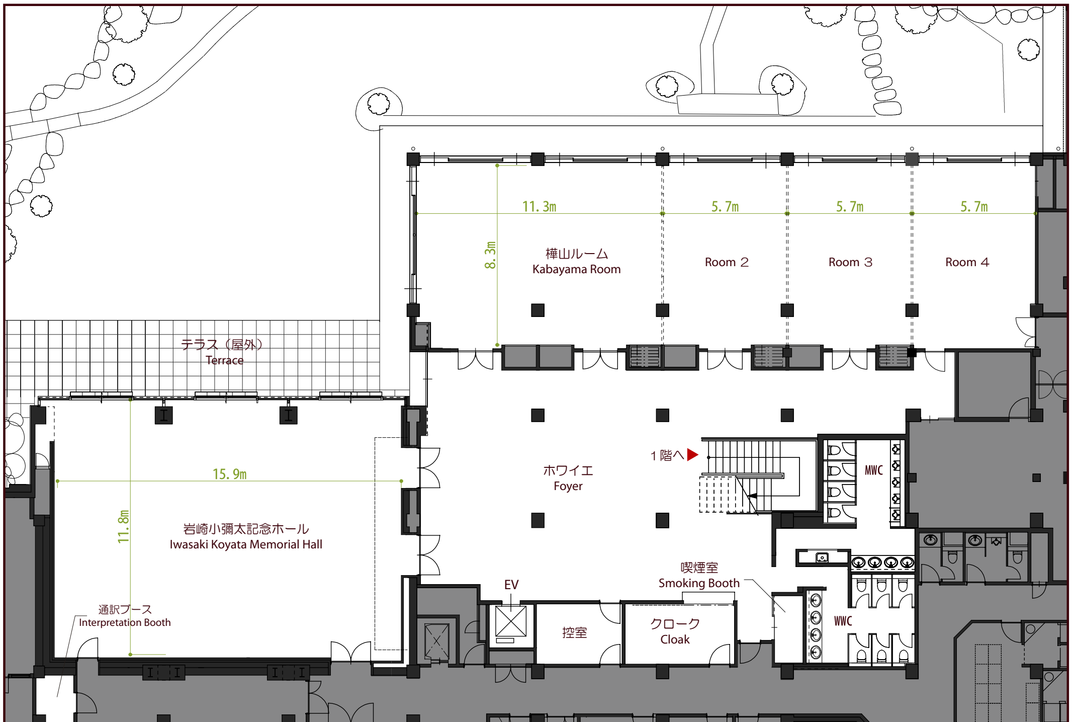
地下宴会場・ホール平面図
